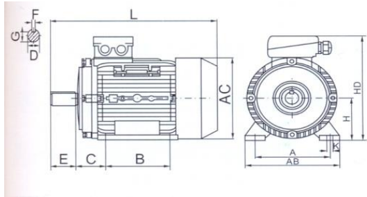
IMB3
