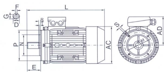
IMB14
