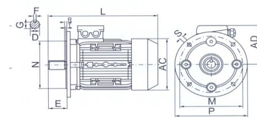
IMB5
