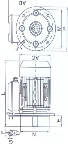
IMB5
