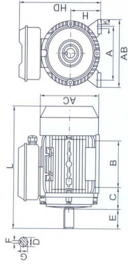
IMB3
